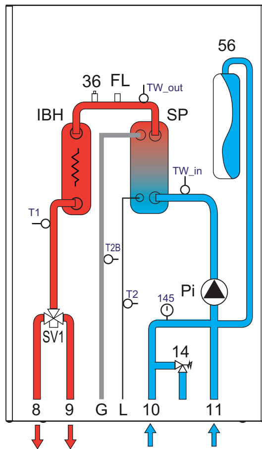
fig. 5 - Hydraulisch schema binnenunit
