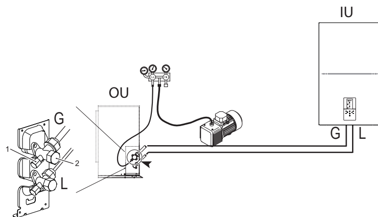
fig. 13 - Luchtzuivering met vacuümpomp
