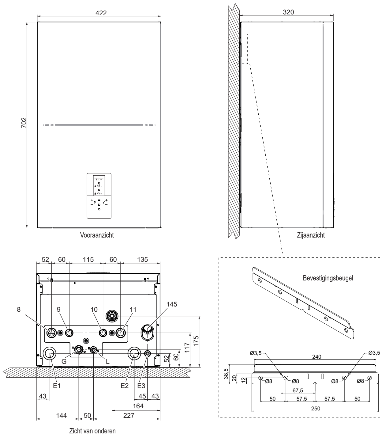
fig. 3 - afmetingen en verbindingen
